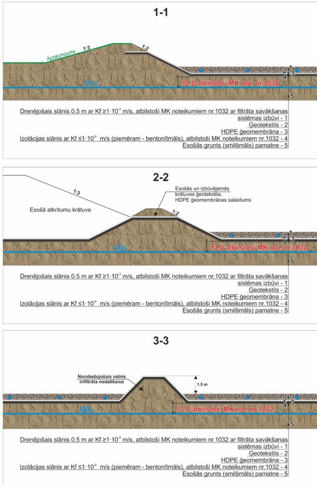
6. attēls. Atkritumu apglabāšanas krātuves uzbūve un tās pievienojums pie esošās krātuves (shematisks zīmējums), 2. alternatīva
