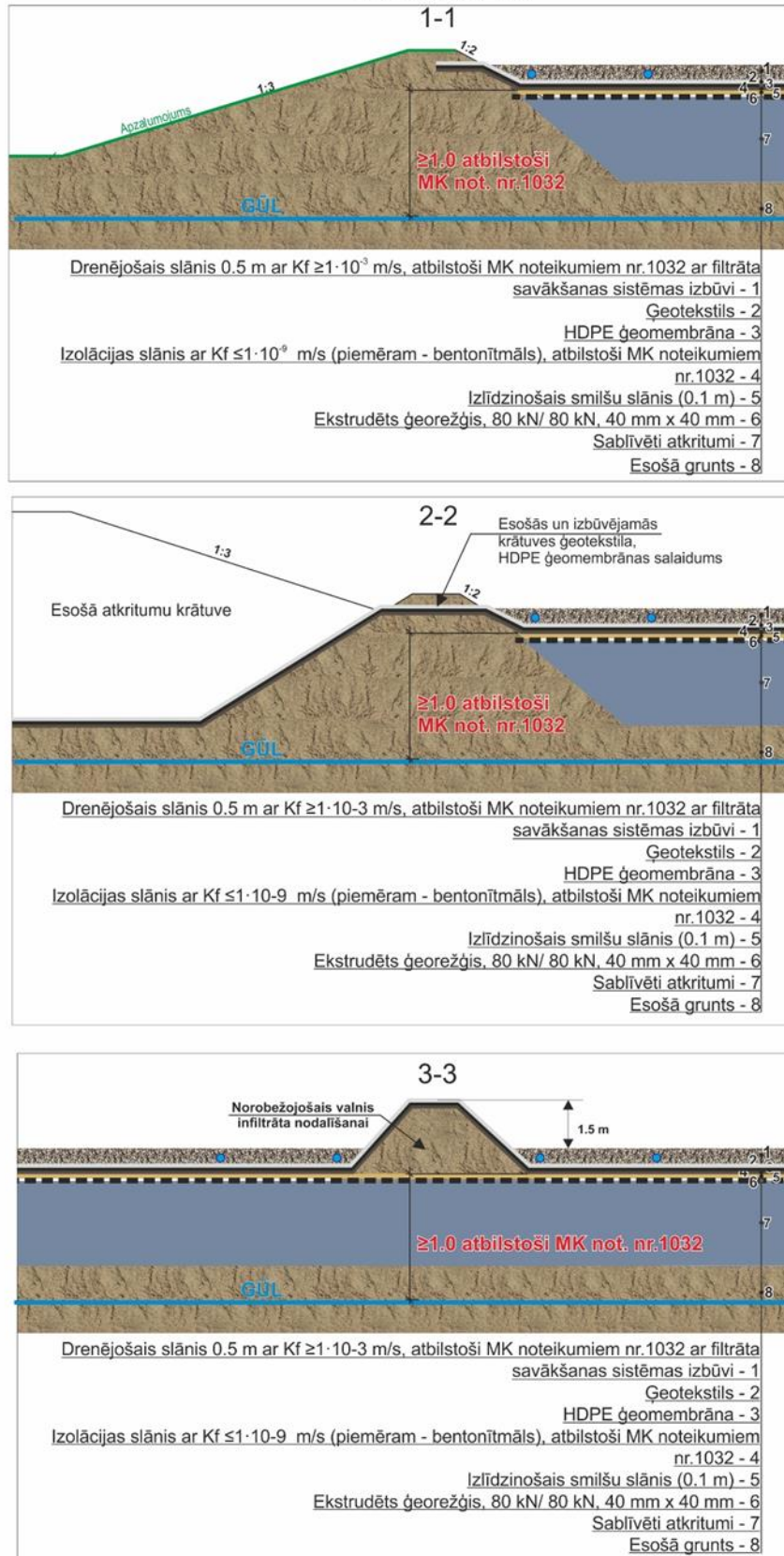
5. attēls. Atkritumu apglabāšanas krātuves uzbūve un tās pievienojums pie esošās krātuves (shematisks zīmējums), 1. alternatīva
