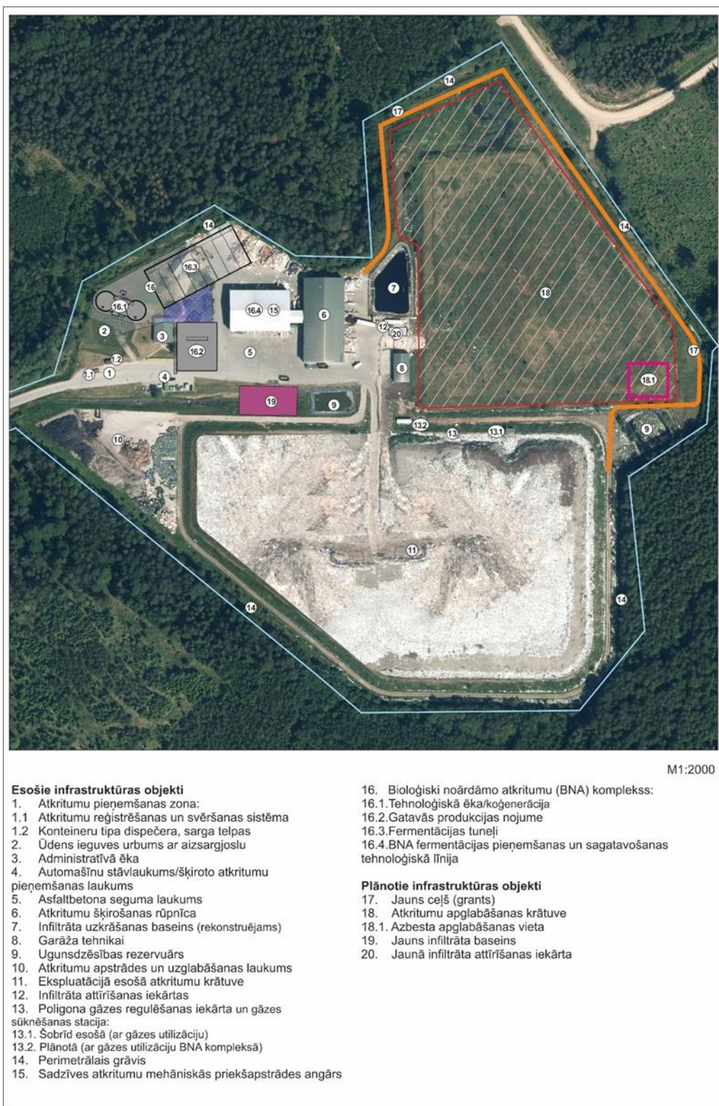
2. attēls. Infrastruktūras objektu izvietojums sadzīves atkritumu poligonā "Janvāri"
