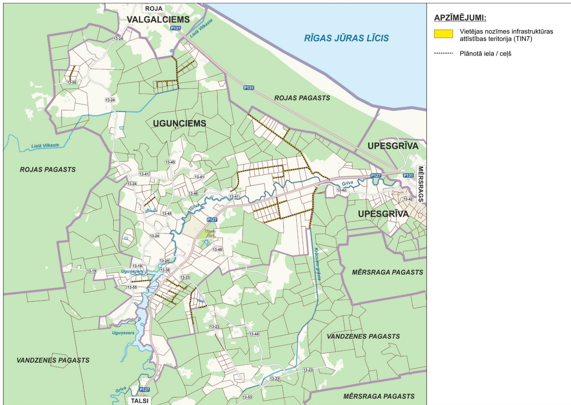
5.attēls. Plānotās ielas / ceļi un pievienojuma vietas valsts autoceļam P127 Uguņciemā
